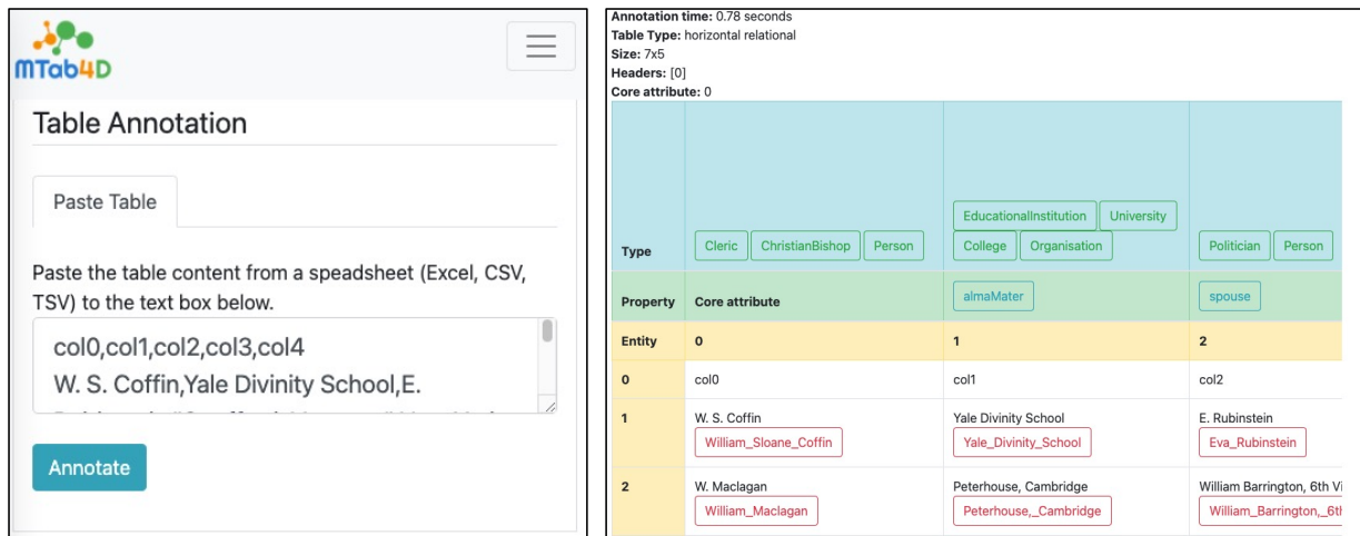
Fig. 8. MTab4D table annotation interface
