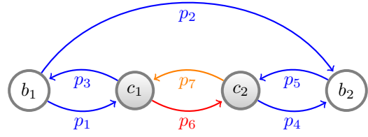
Fig. 10. Counterexample 2
